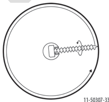
Figure C-2. Center pivot auger (Gislerud et al. 1988).
